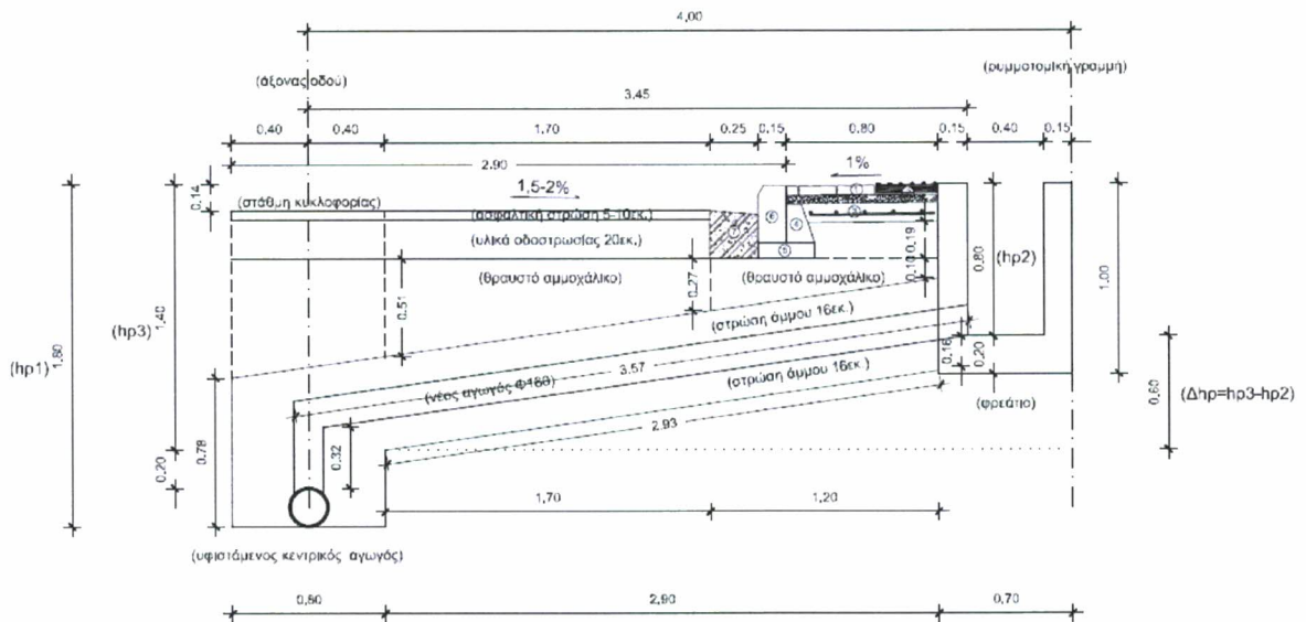
Λ3. ΤΥΠΙΚΗ ΔΙΑΤΟΜΗ ΠΑΡΟΧΕΤΕΥΣΕΩΣ ΣΕ ΥΦΙΣΤΑΜΕΝΗ ΑΣΦΑΛΤΟΣΤΡΩΜΕΝΗ ΟΔΟ ΜΕ ΠΕΖΟΔΡΟΜΙΟ ΜΕΣΟΥ ΠΛΑΤΟΥΣ 8μ.
