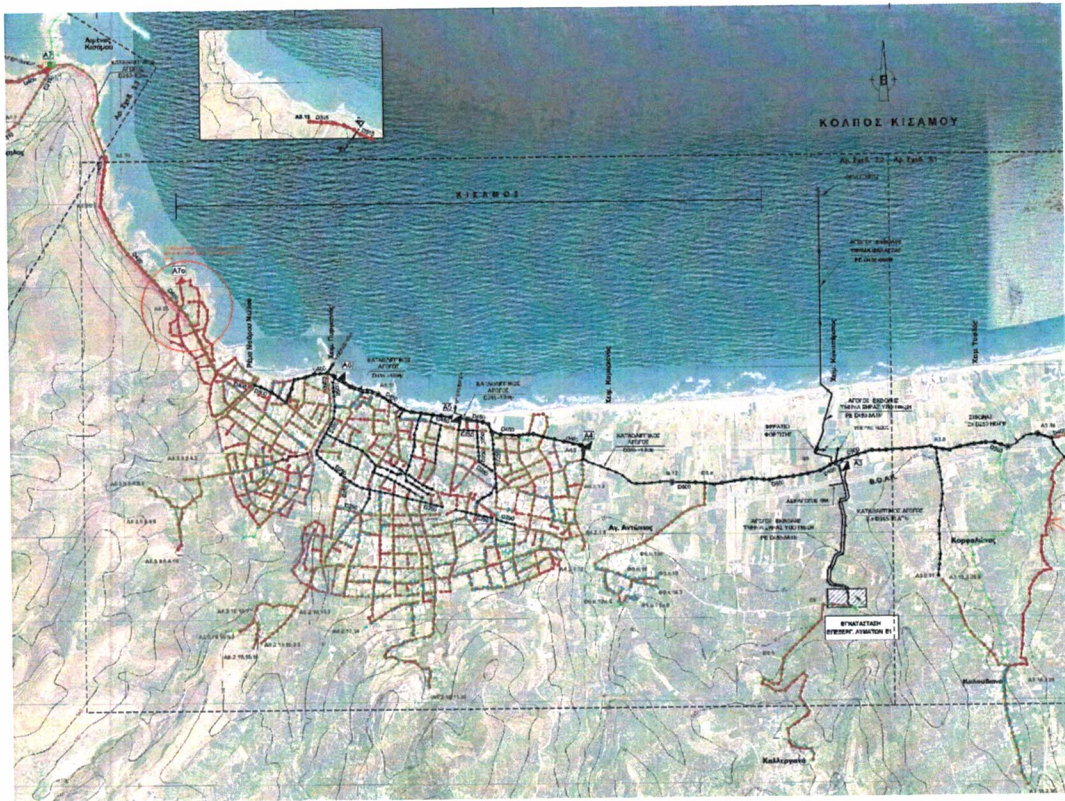
2. Δίκτυο Βιολογικού στην πόλη του Καστελίου κ προς οικισμούς Καλλεργιανά και Καλουδιανά
